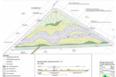
Abbildung 4: Planung dritter Bauabschnitt © Wasser- und Bodenverband der Mittleren Niers
